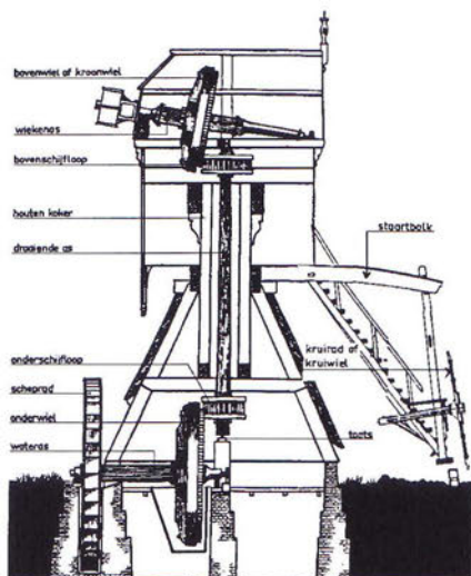
Fig.3. Constructie van de wipmolen (naar Stokhuyzen, Molens)
